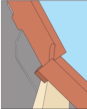
Asenna JP-koukku ja tarkista, että kiinnike on kunnolla kiinni ruoteen takana.
