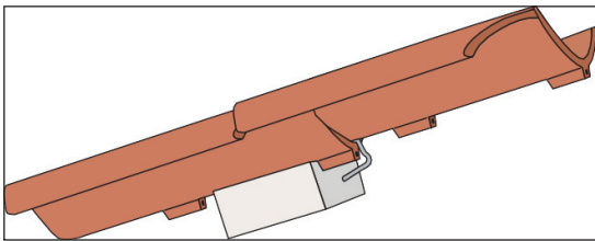
U-tiilikoukkuja käytetään useimmiten alimmassa tiilirivissä ja kaikissa paikoissa, joihin JP-koukkuja ei voida asentaa.
