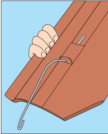
JP-tiilikoukku työnnetään alakautta kannattimen reikään.
