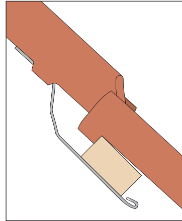
JP-koukku on työnnettävä kokonaan kiinnityskannattimen alta sisälle ja asetettava ruoteen takaosaa vasten siten, että taitteen ja ruoteen alareunan väliin jää tilaa.
