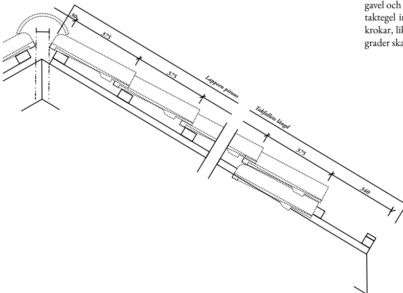
Kiinnitys tiilikitiinnikkeillä. Fästning med tegelkrok.
