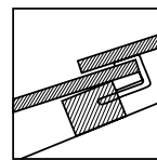
Kiinnitys tiilikitiinnikkeillä. Fästning med tegelkrok.
